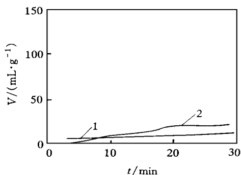
图 11 硬脂酸用量对发泡剂 AC 热分解特性的影响(170) 1—0份;2—0.25份
