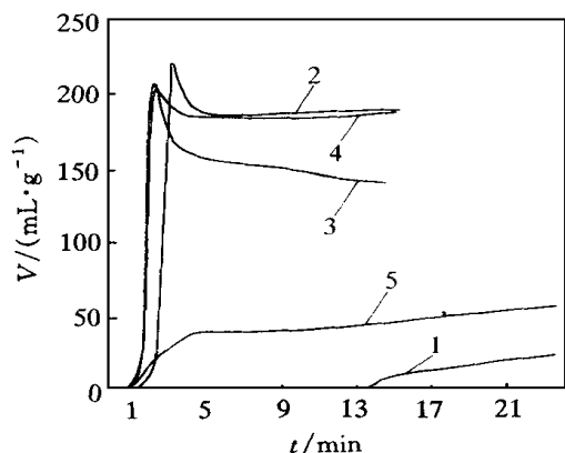
图4 硬脂酸钡对发泡剂AC热分解特性的影响(170 )
