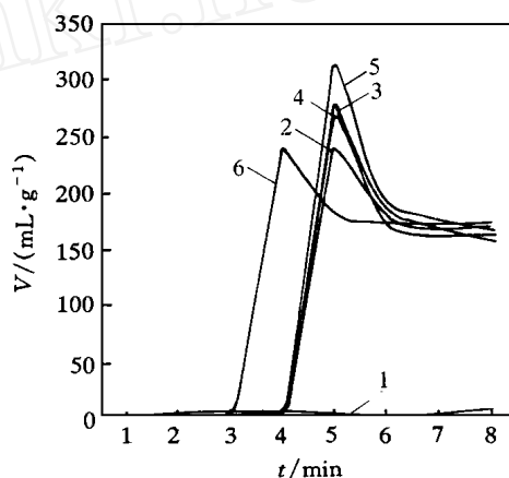
图5 氧化锌用量对发泡剂AC热分解特性的影响(170 )
