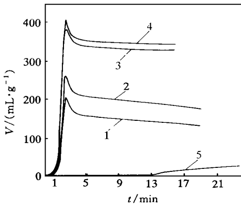
图 2 二盐用量对发泡剂 AC 热分解特性的影响 (170 )
