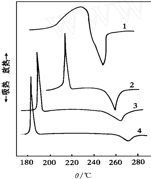
图 7 不同配比的发泡剂 AC/氧化锌的 DSC 曲线 配比:1—1/0;2—1/0.02;3—1/0.04;4—1/0.10
