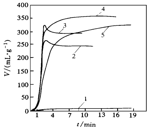
图 8 柠檬酸用量对发泡剂 AC 热分解特性的影响(170 )
