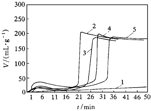
图 12 柠檬酸钠用量对发泡剂 AC 热分解特性的影响(170 )
