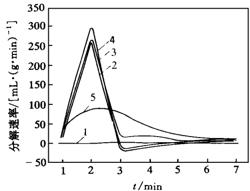
图 9 柠檬酸用量对发泡剂 AC 分解速率的影响(170 )
