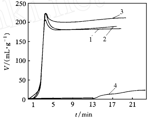
图 3 硬脂酸铅用量对发泡剂 AC 热分解特性的影响(170 )
