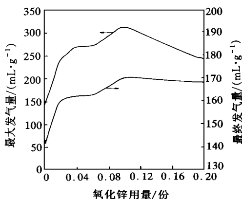
图6 氧化锌用量对发泡剂AC发气量的影响(170 )
