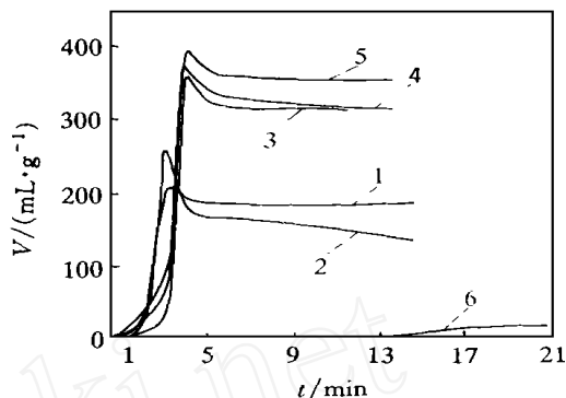
图 1 三盐用量对发泡剂 AC 热分解特性的影响(170 ^\circ\text{C} )
